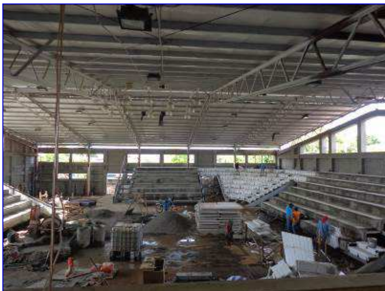
Vista interna de las instalaciones del Gimnasio de Boxeo, donde se aprecia la instalación de la estructura metálica principal y covintec de graderías costado Norte, Noreste y Este
